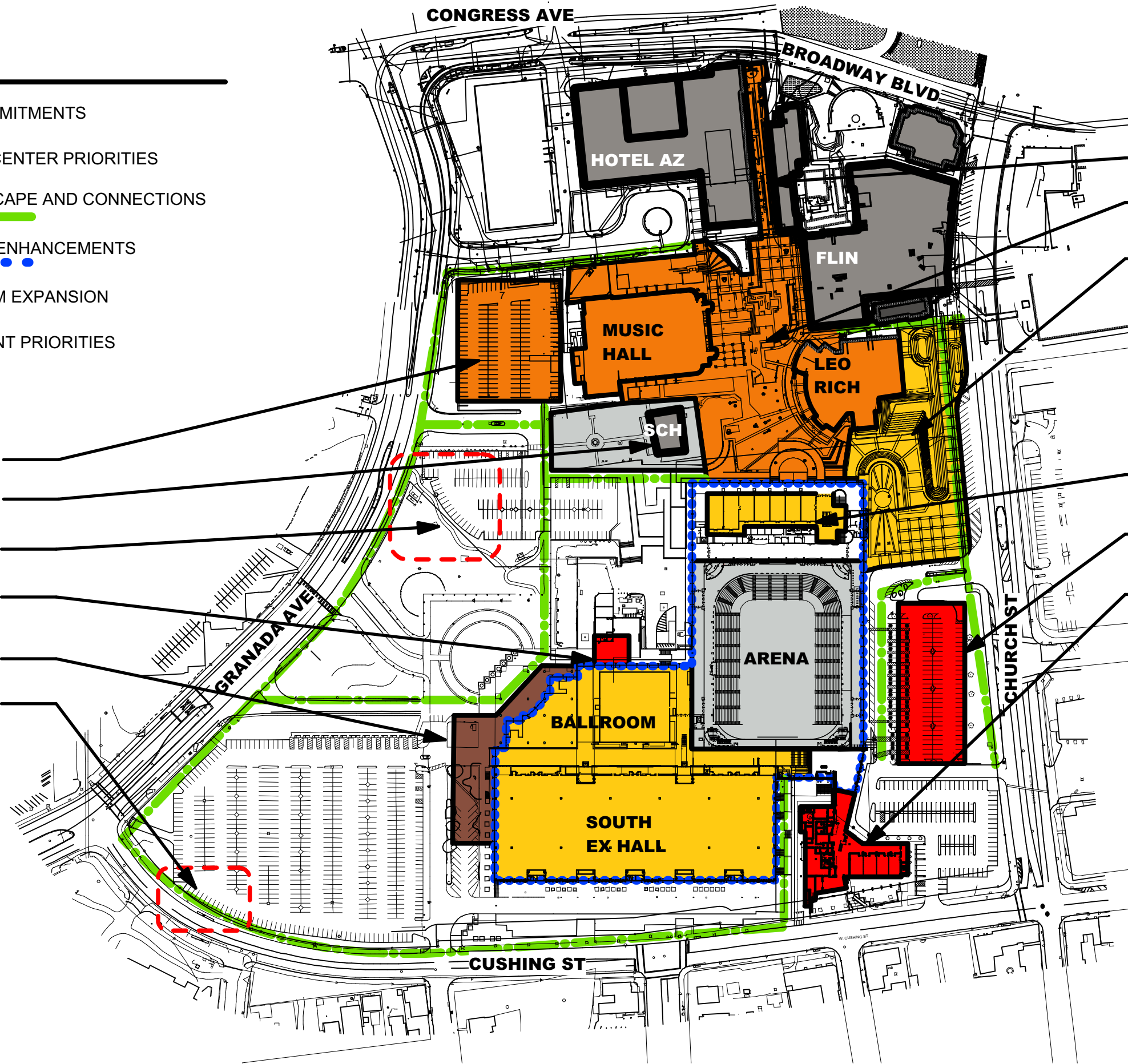
TCC SITE PLAN
